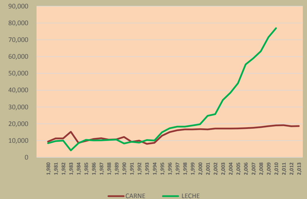
PRODUCCION CARNE Y LECHE DE VACUNOS (TM) 1980 -2013
