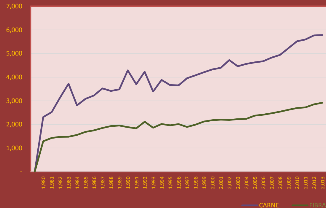
PRODUCCION CARNE Y FIBRA DE ALPACA (TM) 1980 -2013
